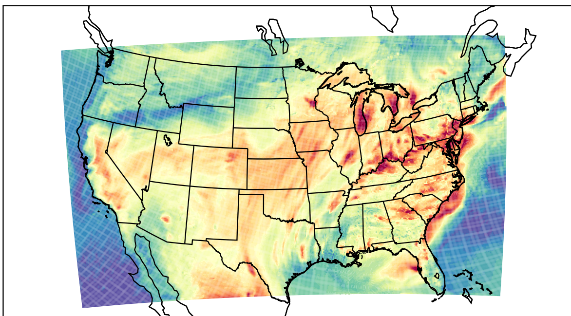
WRF (2019-07-18_22:00:00)
