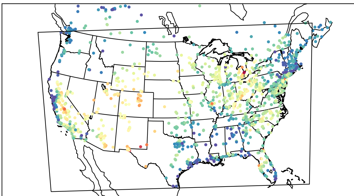
AirNOW (2019-07-18_18:00:00)
