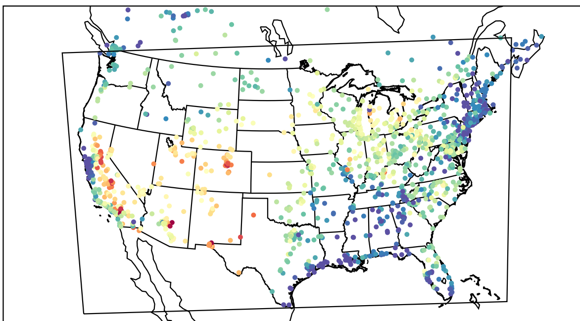
AirNOW (2019-07-18_23:00:00)
