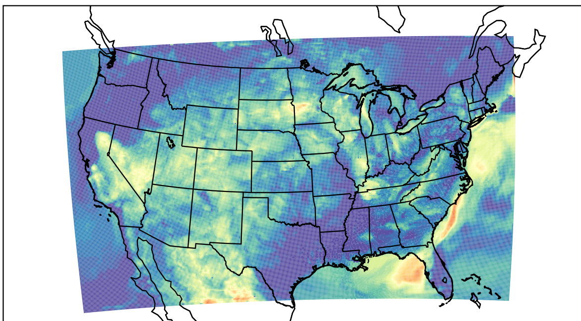
WRF (2019-07-18_11:00:00)
