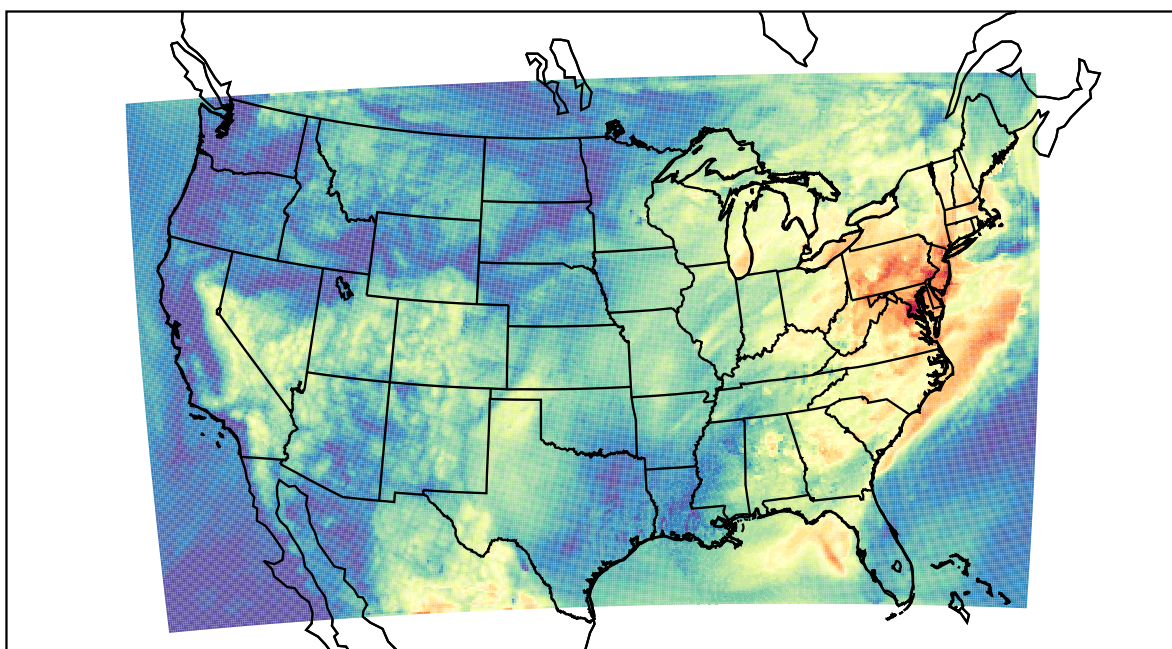
WRF (2019-07-19_14:00:00)
