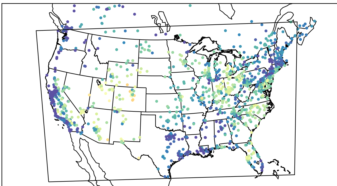
AirNOW (2019-07-18_15:00:00)
