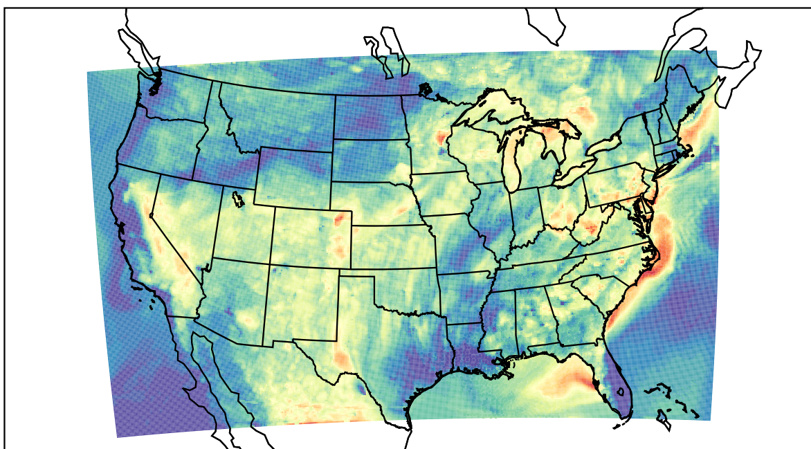
WRF (2019-07-19_04:00:00)
