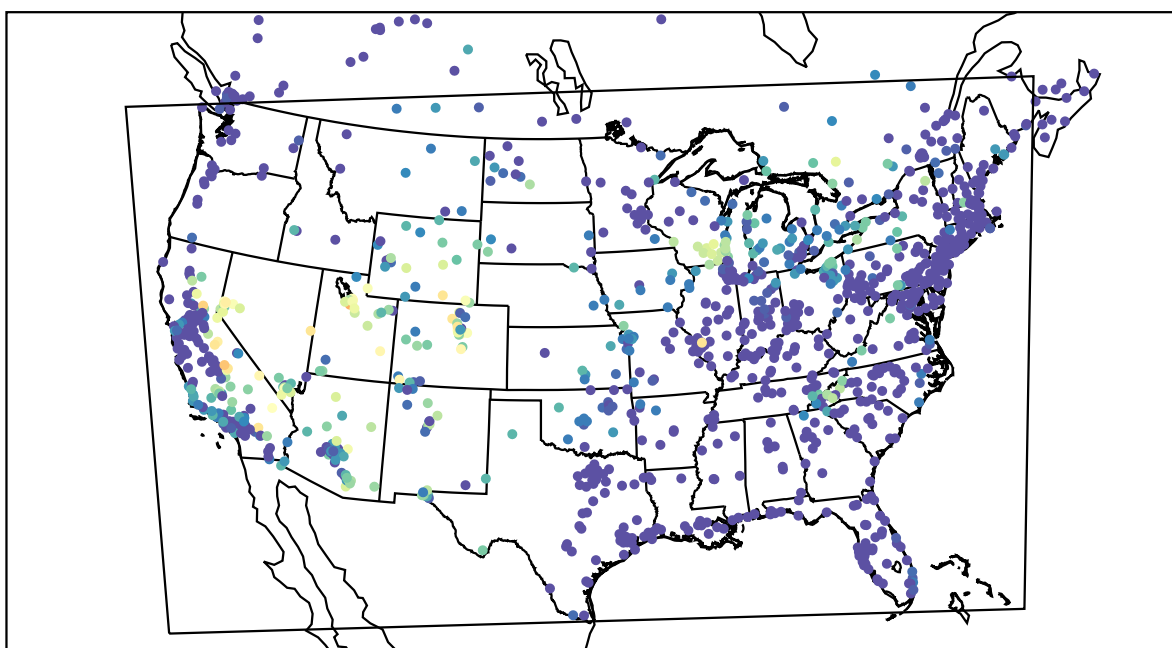
AirNOW (2019-07-19_10:00:00)
