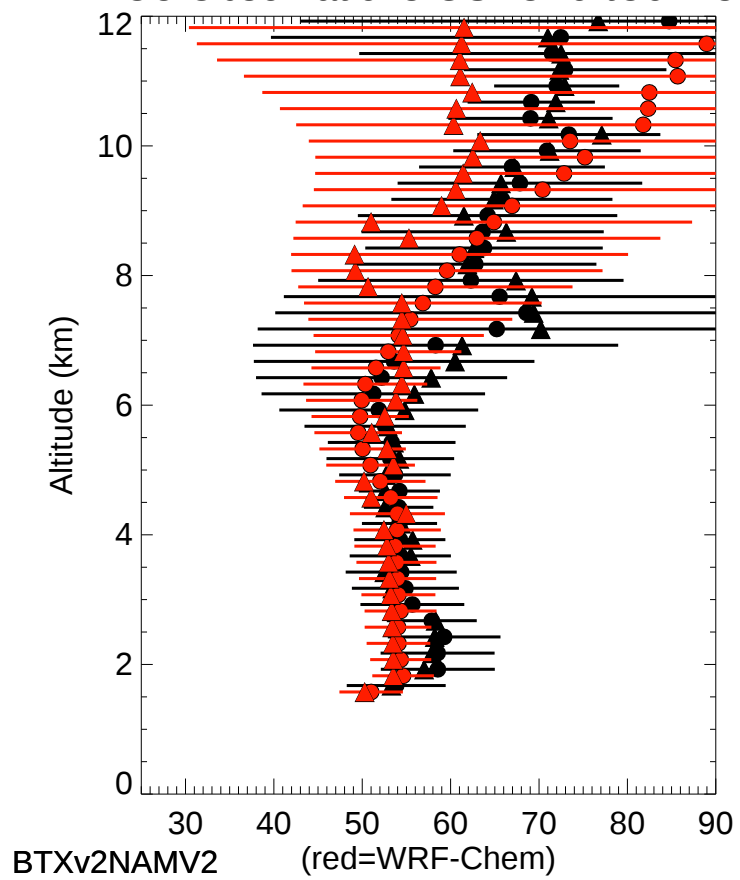
O3 Observations GSFCFortCollins
