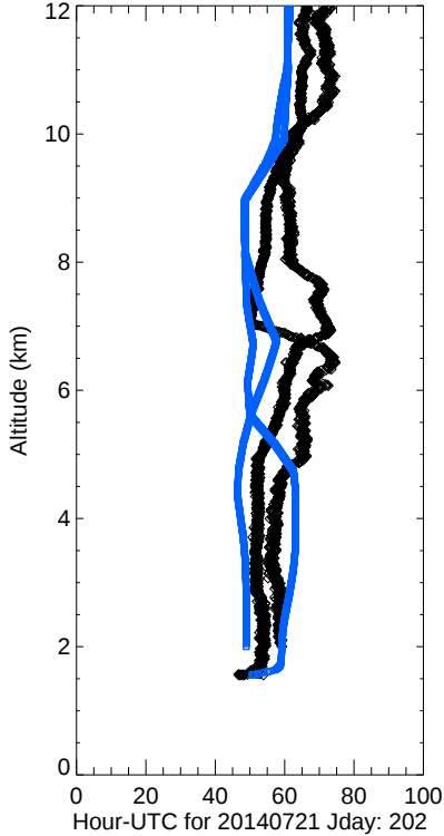
O3 Observations GSFCFortCollins
