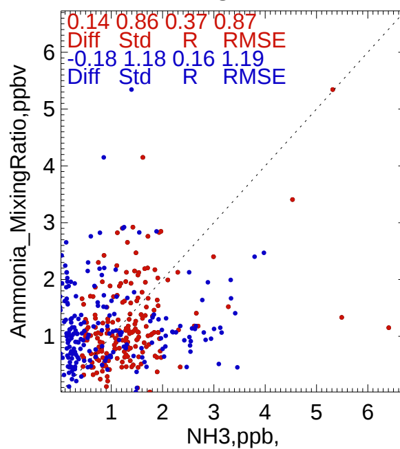
> 3 km
