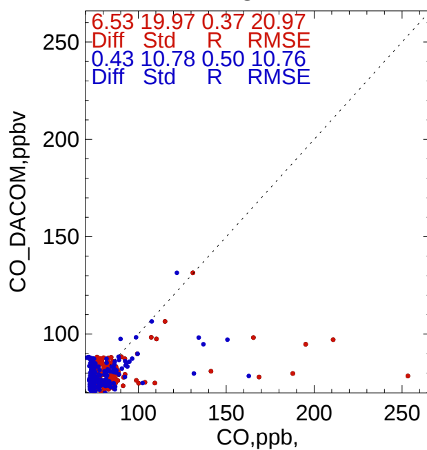
> 3 km
