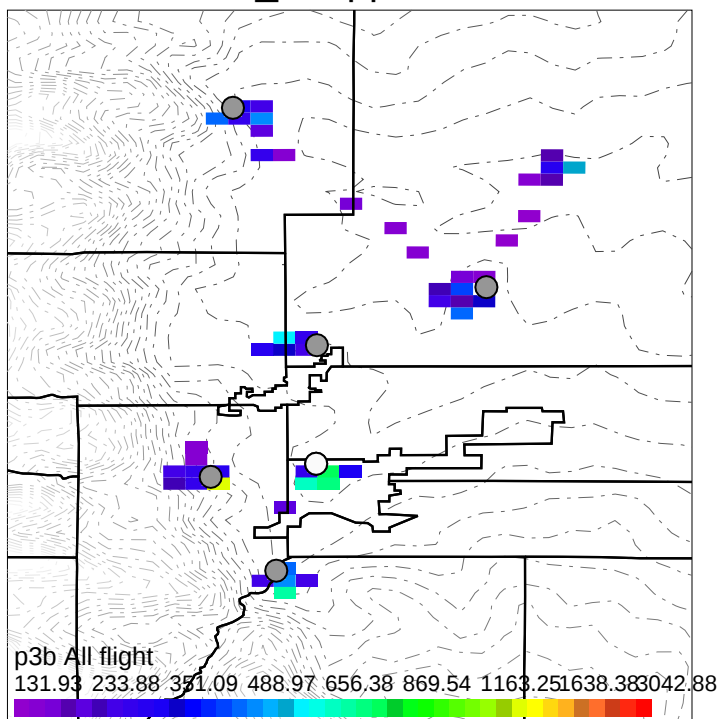
HNO3_LIF,pptv > 3 km
