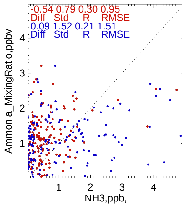
> 3 km
