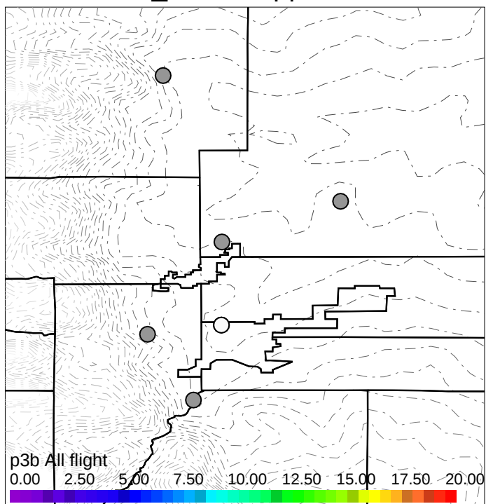
Ethane_TILDAS,ppbv > 3 km
