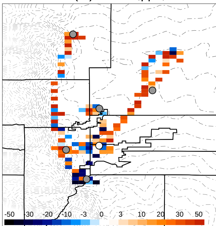
Model-Obs(%) HCHO,ppb, &lt; 3 km
