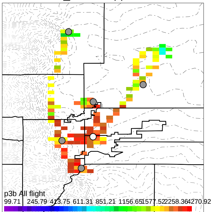
Model-Obs(%) HCHO,ppb, &lt; 3 km
