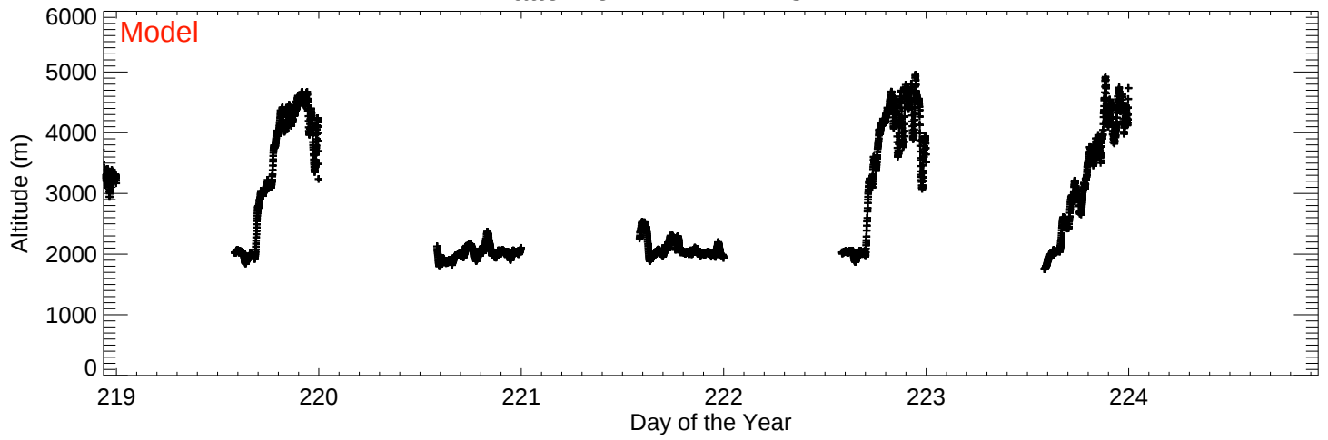
PlattevilleMPL
