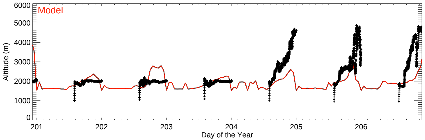
PlattevilleMPL BTXv2ECMWFRAp
