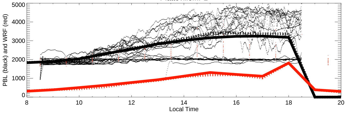
PlattevilleMPL
