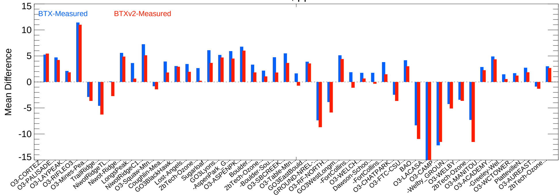
O3, ppb
