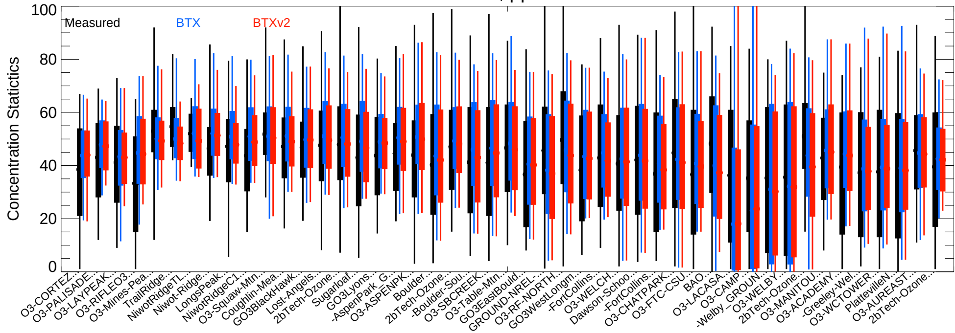
O3, ppb
