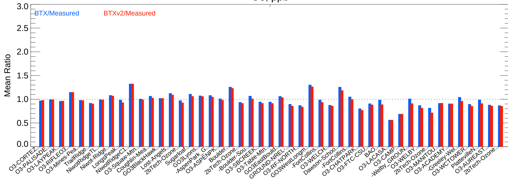
O3, ppb
