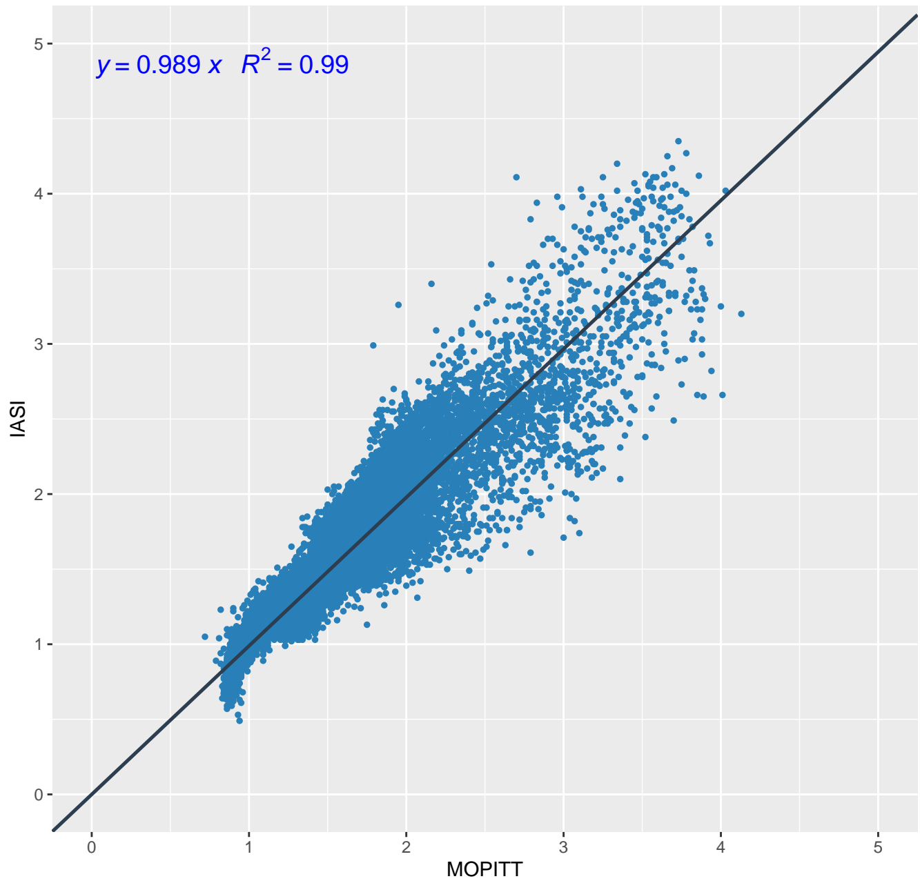
MOPITT IASI over land (Sep)
